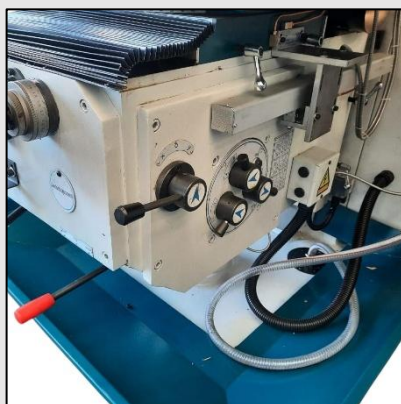
Caja de avances y bajada automática de husillo
